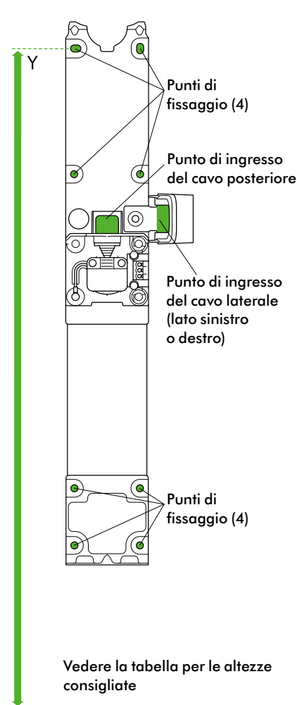
Piastra posteriore
